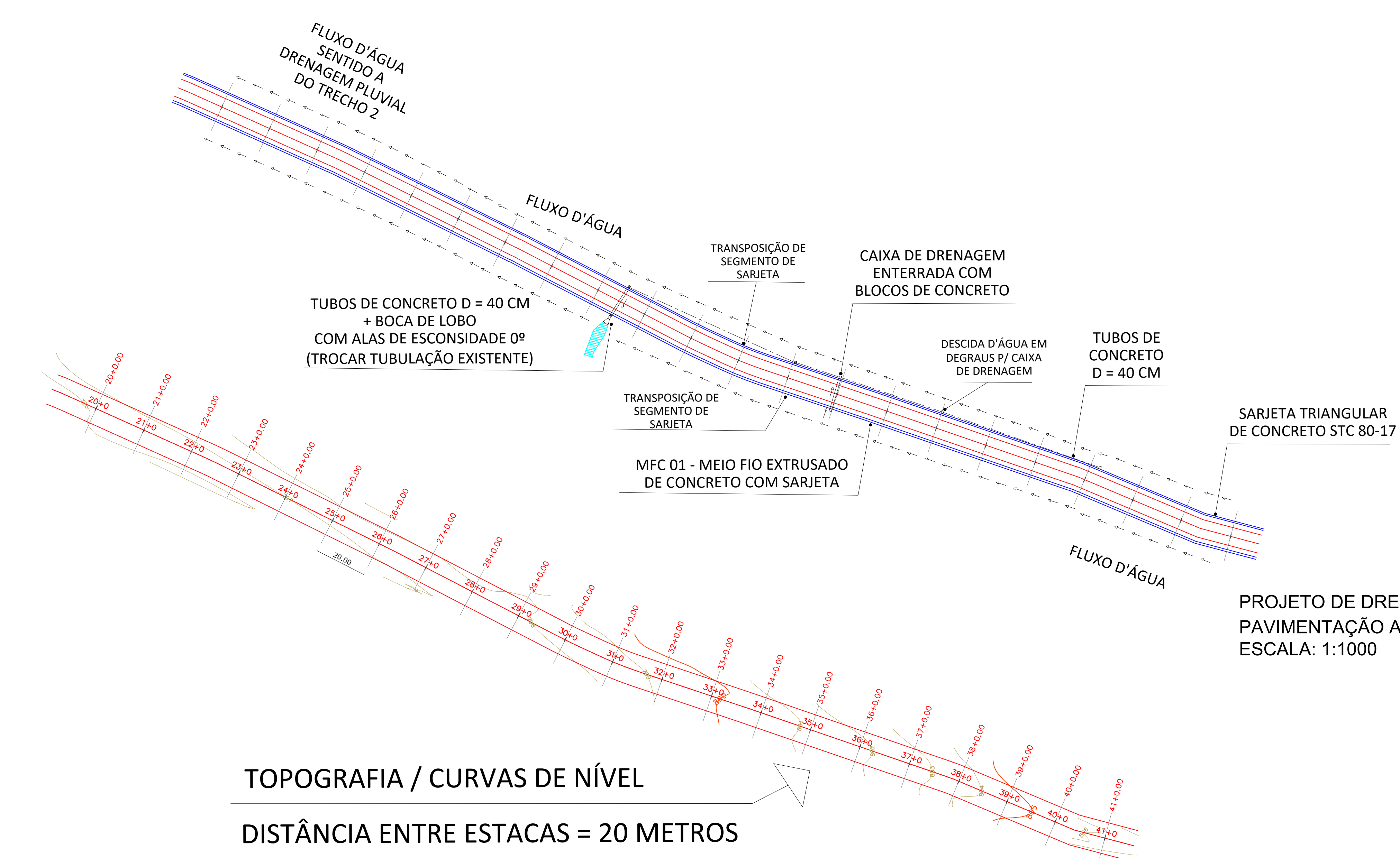
PROJETO TOPOGRÁFICO CURVAS DE NÍVEL EM METROS ESCALA 1:1000
