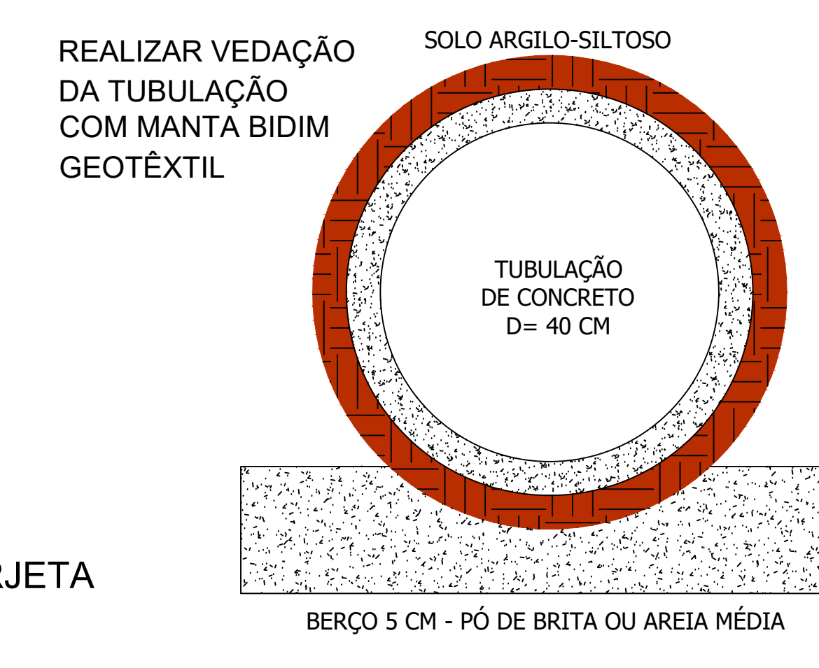
DETALHAMENTO TUBOS DE CONCRETO EM CM SEM ESCALA
