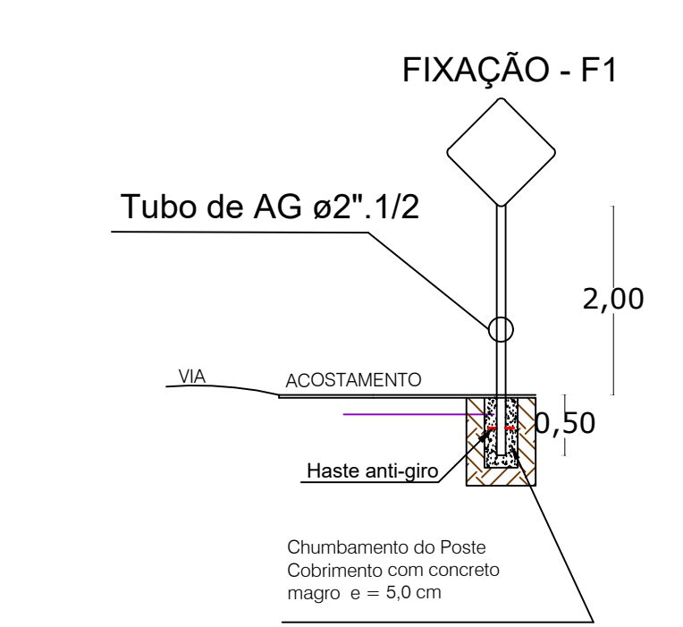
DETALHES FIXAÇÃO DE PLACAS SEM ESCALA
