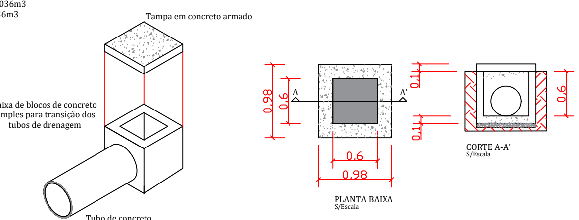
DETALHES CAIXAS DE DRENAGEM ESCALA 1:50
