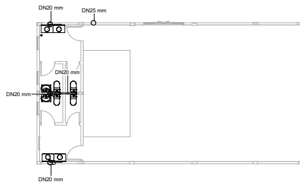
2 PLANTA DE PISO 1 : 100
