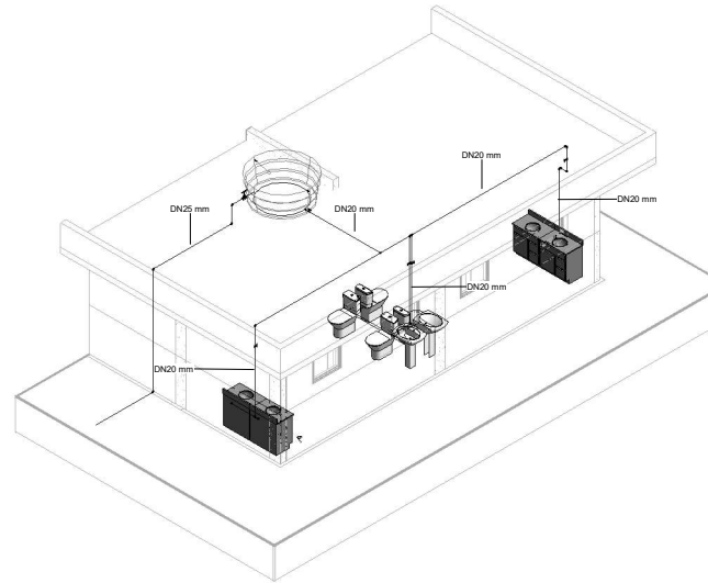
3 ISOMETRICO
