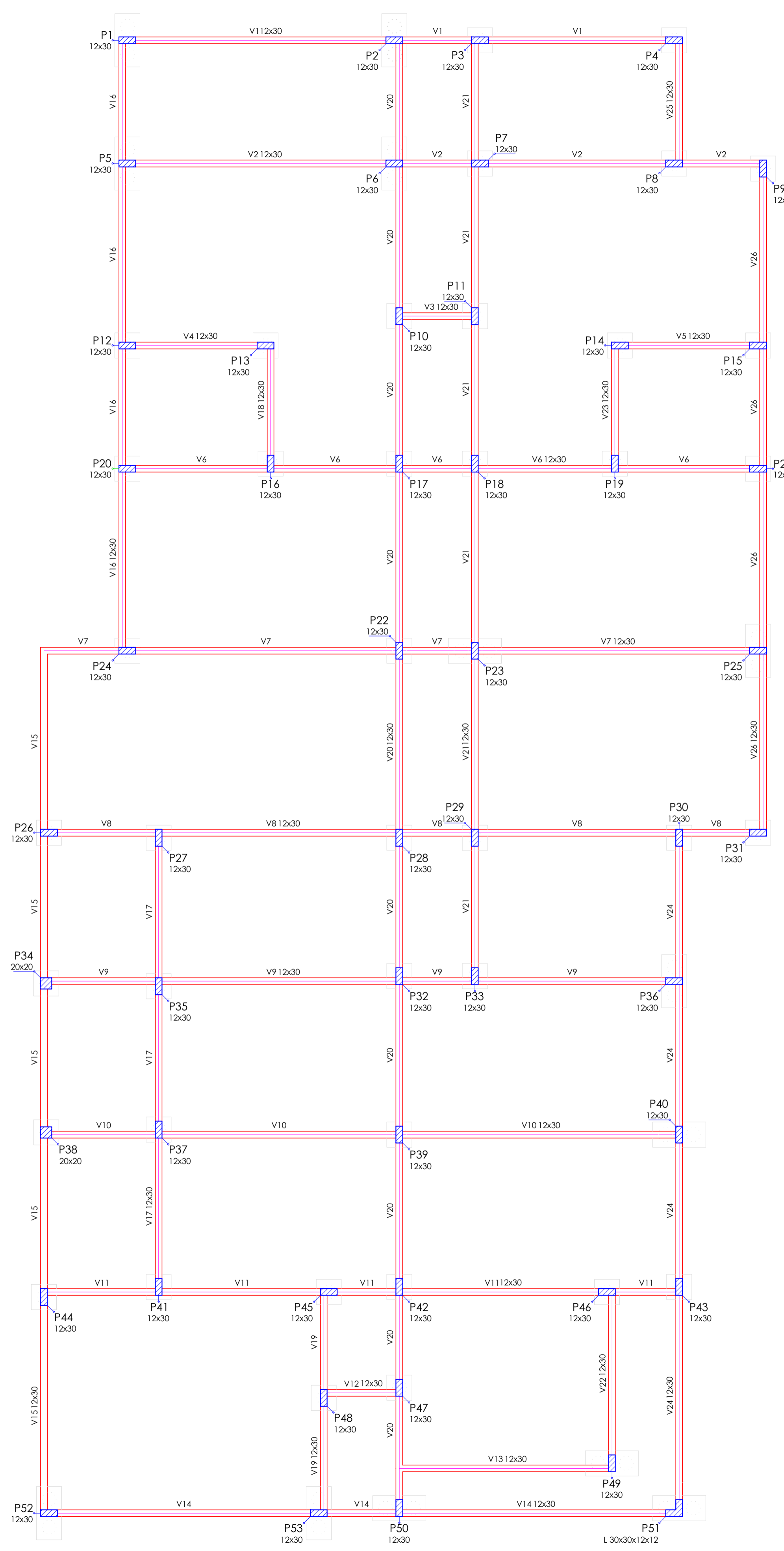
Forma do pavimento Fundações (Nível 20) escala 1:50
